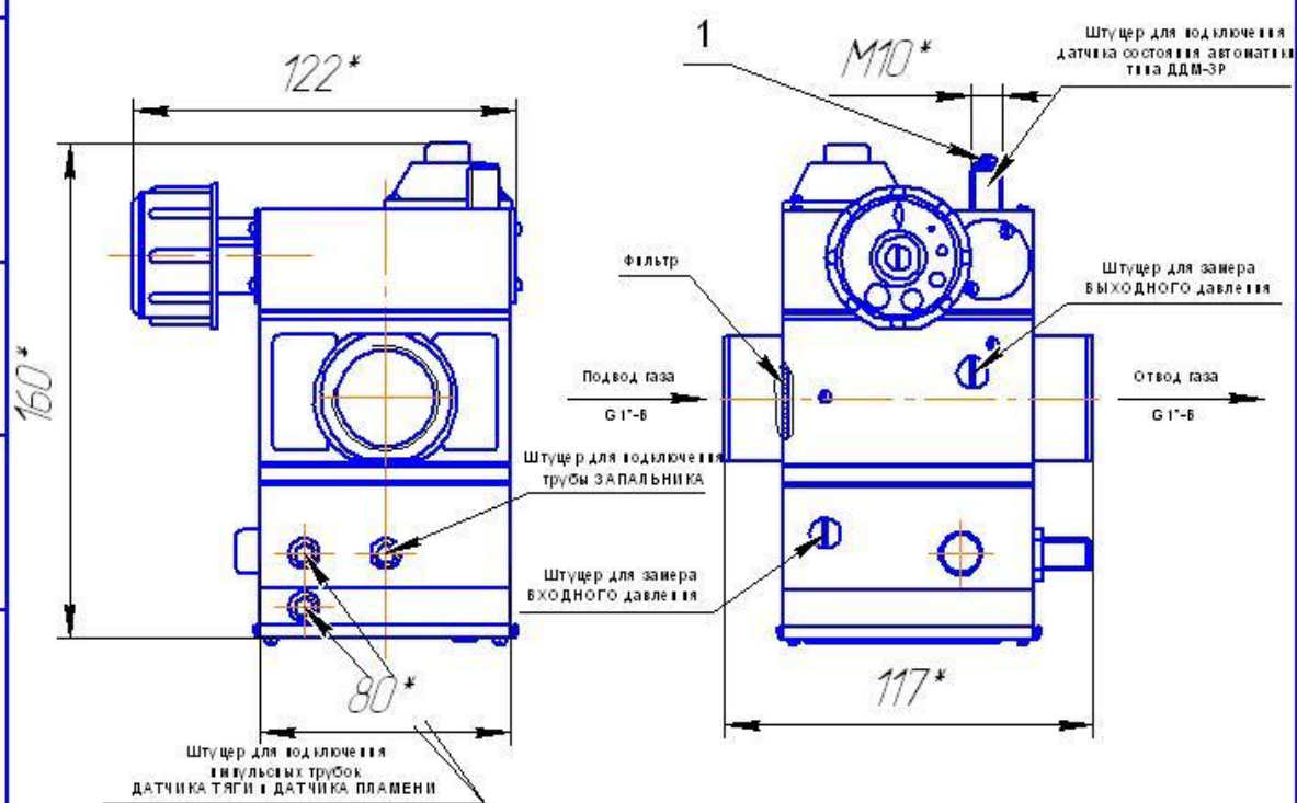
Рис.2Б Схема расположения точек подключения блока автоматики.
